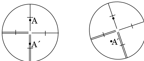
Коллимационная ошибка
